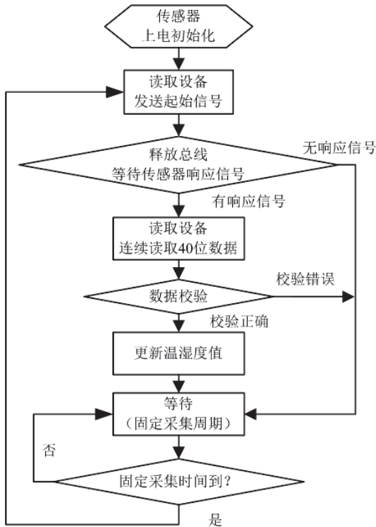
图11: 单总线读取流程图
