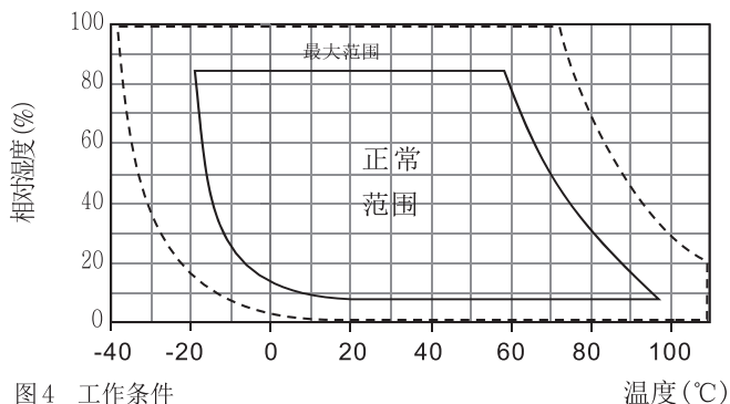
图4 工作条件
